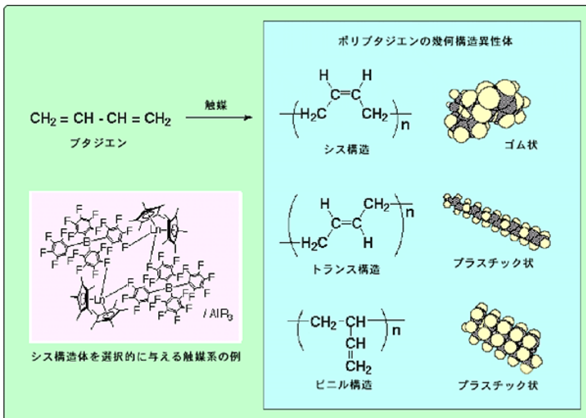
図1 ブタジエンの幾何構造異性体
