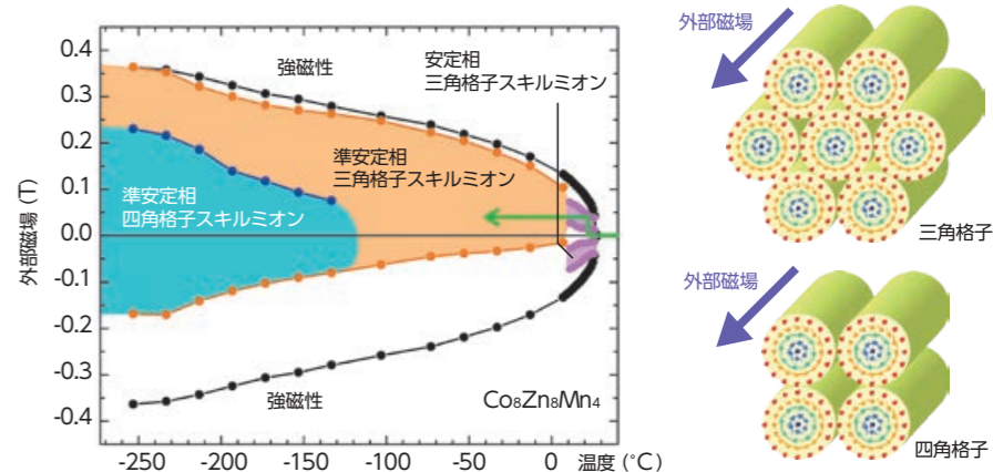
図2 室温を含む広い温度・磁場領域に存在するスキルミオン Co_8Zn_8Mn_4 において、22℃・外部磁場0.04T(テスラ)で安定相スキルミオン三角格子を生成した後、外部磁場をかけたまま冷却した(緑色の矢印)。すると、広い温度・磁場領域で準安定相スキルミオンが存在し続け、さらに低温では四角格子に構造が変化した。
