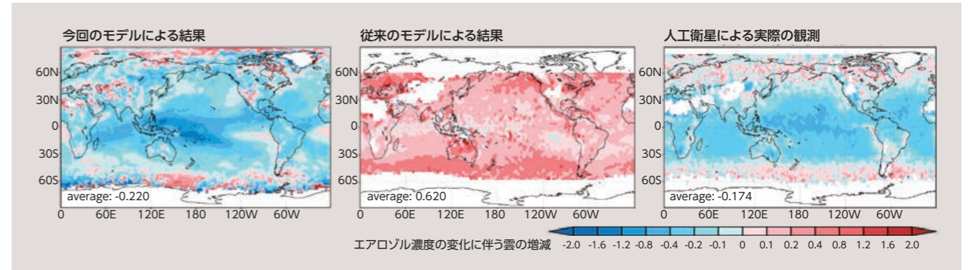
図5 エアロゾル濃度の変化に伴う雲の量の変化 赤色はエアロゾルの増加に伴って雲が増加する領域を示し、青色はエアロゾルが増加すると雲が減少する領域を示す。近年、大気中のエアロゾル濃度は増加している。人工衛星による実際の観測では、雲が減った領域が多い(右)。従来の低解像度シミュレーションでは、ほとんどの領域でエアロゾルが増えると雲が増えることを示す計算結果となっていた(中央)。今回の高解像度シミュレーションでは、観測と同様にエアロゾルが増えたときに雲が減る領域が多いことが示されている(左)。
