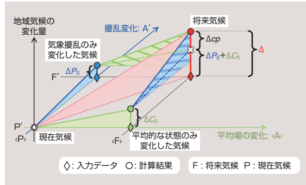
図2 地域気候の変動を理解する新評価手法 地域気候の変化は現在の気候と将来の気候の差( \Delta )で表される。現在気候から地球全体の平均的な状態のみ変化した場合の地域気候変化は \Delta C_0 、現在気候から台風や温帯低気圧といった気象擾乱のみ変化した場合の地域気候変化は \Delta P_0 で表される。その二つの変化から推測される将来変化は \times 印であり、実際の将来気候(赤丸)と異なる。この差が、地球全体の平均的な状態の変化と気象擾乱の変化の相互作用による変化( \Delta cp )である。
