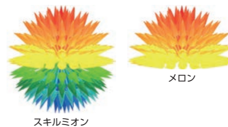
図8 スキルミオンとメロンのトポロジー トポロジーは連続変形を行っても変化しない量(トポロジカル数)を用いて、形を分類する理論である。スキルミオンをつくる電子スピンの矢印の始点を1点に集めると、終点は全球を覆うようにあらゆる方向を向く。そのトポロジカル数は-1である(左)。電子スピンの内向きの反スキルミオンのトポロジカル数は+1。 一方、メロンの電子スピンの矢印の終点は全球ではなく半球だけを覆い、トポロジカル数は-1/2(右)。アンチメロンは電子スピンの内向向きで、トポロジカル数は1/2である。
