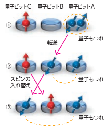
図 隣り合わない量子ビット間で量子もつれをつくる手順 ①量子ビットAに2個の電子を入れて量子もつれをつくる。 ②そのうちの1個の電子を量子ビットBに転送する。 ③量子もつれの関係にない量子ビットCとBのスピンを入れ替える。こうして、隣り合っていない量子ビットAとCの量子もつれを実現できる。
