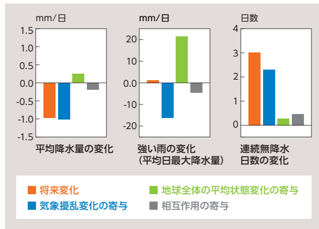
図3 上記手法によるデモンストレーション計算 西日本を中心とする領域に対して、6～9月の4カ月について25年分のシミュレーションを行った。平均降水量の将来変化(左)は、気象擾乱の変化(青)の影響が大きく、地球全体の平均的な状態の変化(緑)の影響だけでは説明できない。強い雨の将来変化(中央)は、気象擾乱の変化の影響と地球全体の平均的な状態の変化の影響が打ち消し合っている。連続無降水日数の将来変化(右)は、気象擾乱の変化の影響が大きく、地球全体の平均的な状態の変化の影響だけでは説明できない。
